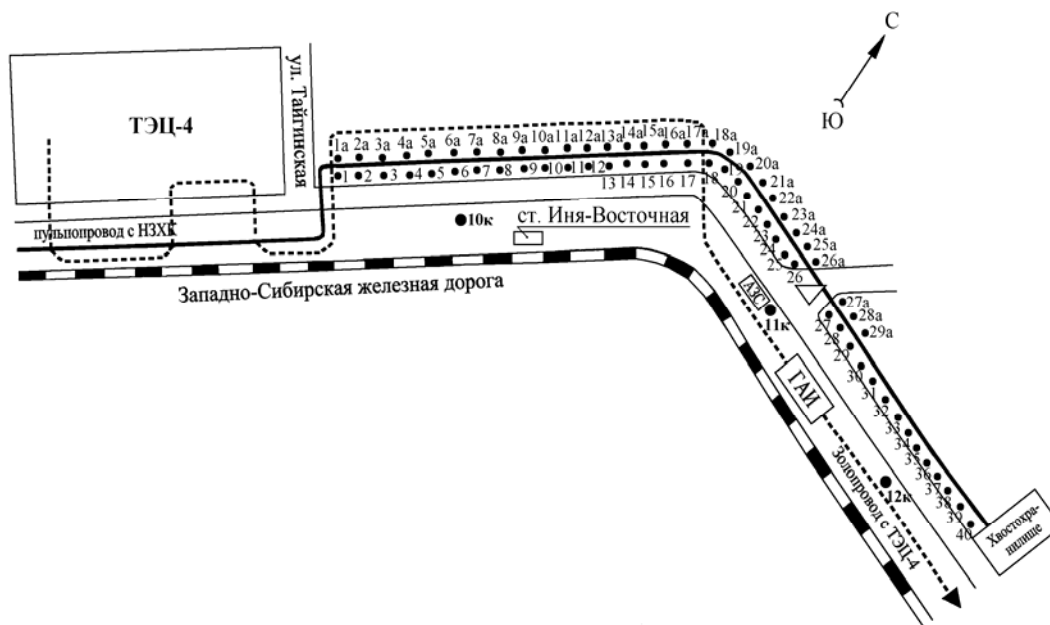
Рис. 2.10. Схема расположения точек контроля радиационной обстановки в районе пульпопровода НЗХК:
