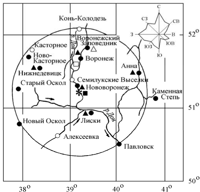
Рис. 4.13. Расположение пунктов радиационного мониторинга в 100-км зоне вокруг НВАЭС:
