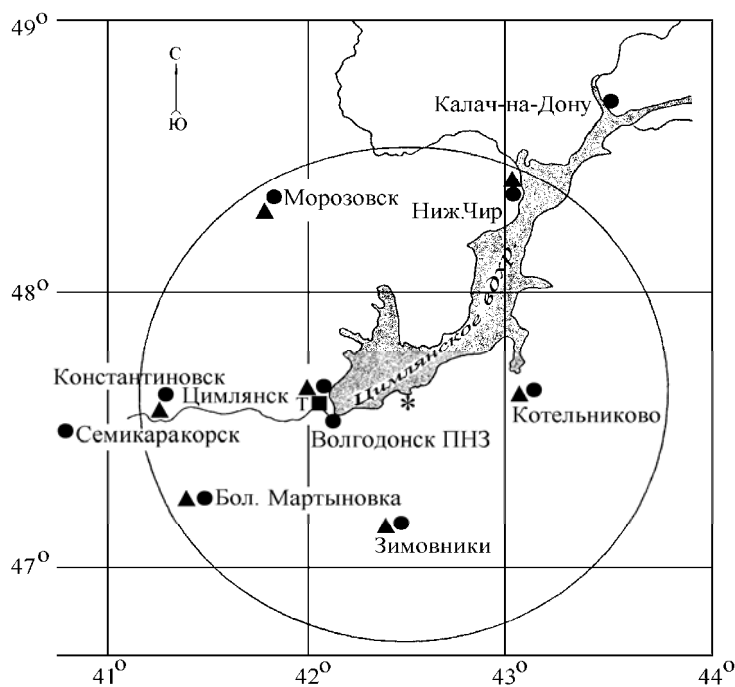
Рис. 4.15. Расположение пунктов радиационного мониторинга в 100-км зоне вокруг Ростовской АЭС:
