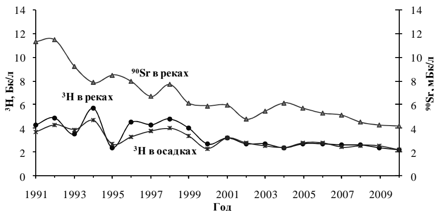
Рис. 1.4. Динамика изменения объемной активности ^3\text{H} в реках, в осадках и ^{90}\text{Sr} в реках на территории РФ
