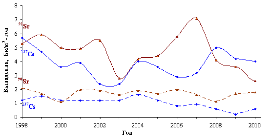
Рис. 5.2. Динамика выпадений радионуклидов на подстилающую поверхность на территории Восточно-Уральского радиоактивного следа:
