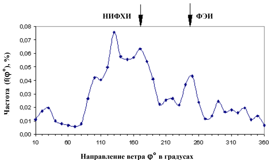
Рис. 3.9. Распределение количества случаев регистрации ^{131}\text{I} от направления ветра в 2009 г.
