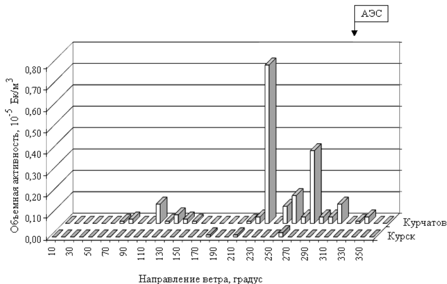
Рис. 4.11. Зависимость средней объемной \gamma -активности техногенных радионуклидов за 2010 г. в атмосферных аэрозолях от преобладающего направления ветра в гг. Курске и Курчатове
