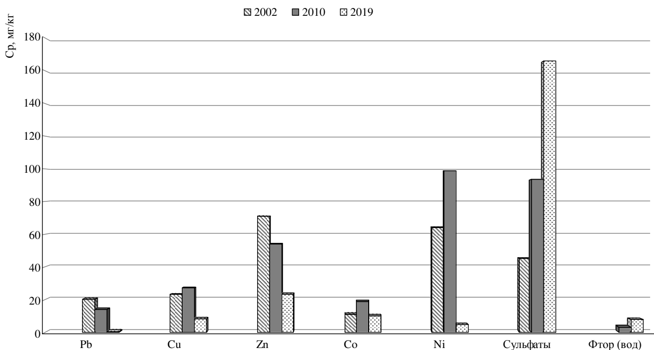
Р и с у н о к 6 – Средние значения массовых долей ТПП в почвах фонового участка в районе г. Усолье-Сибирское Иркутской области в разные годы наблюдений
