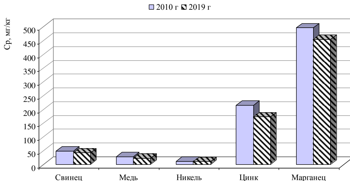
Р и с у н о к 12 – Значения массовых долей валовых форм тяжелых металлов в почве на территории пгг. Славянка в разные годы наблюдений
