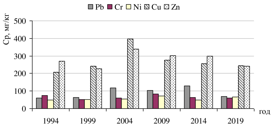
Р и с у н о к 18 – Динамика изменений содержания тяжёлых металлов в почве на территории г. Первоуральска в 1994 – 2019 гг.
