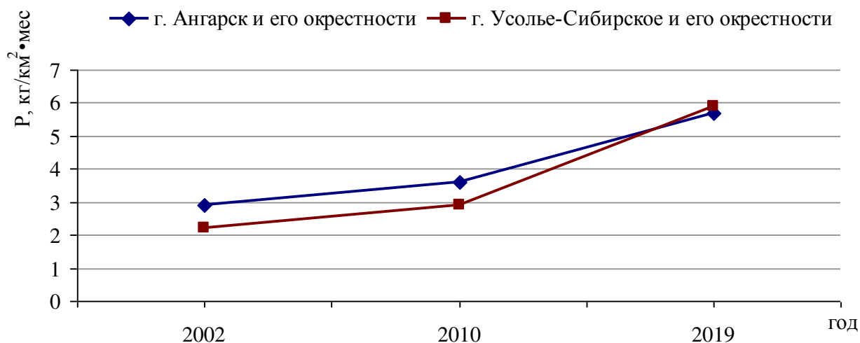
Р и с у н о к 25 – Плотность атмосферных выпадений водорастворимых соединений фтора (P, кг/км 2 ·мес) по данным обследования снежного покрова в городах Ангарск и Усолье-Сибирское Иркутской области в разные годы наблюдений
