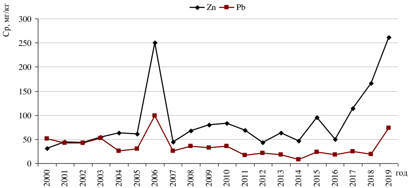
Р и с у н о к 15 – Многолетняя динамика изменений содержания цинка и свинца в почве ПМН г. Томска.
